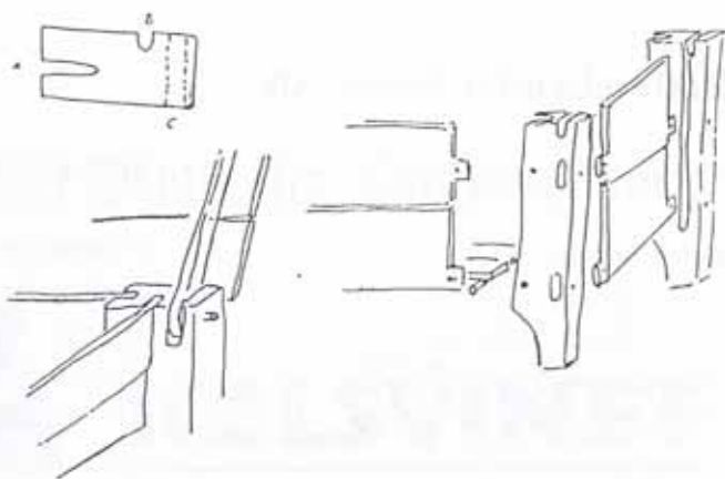
- KONSTRUKTION STOLPEKISTE
